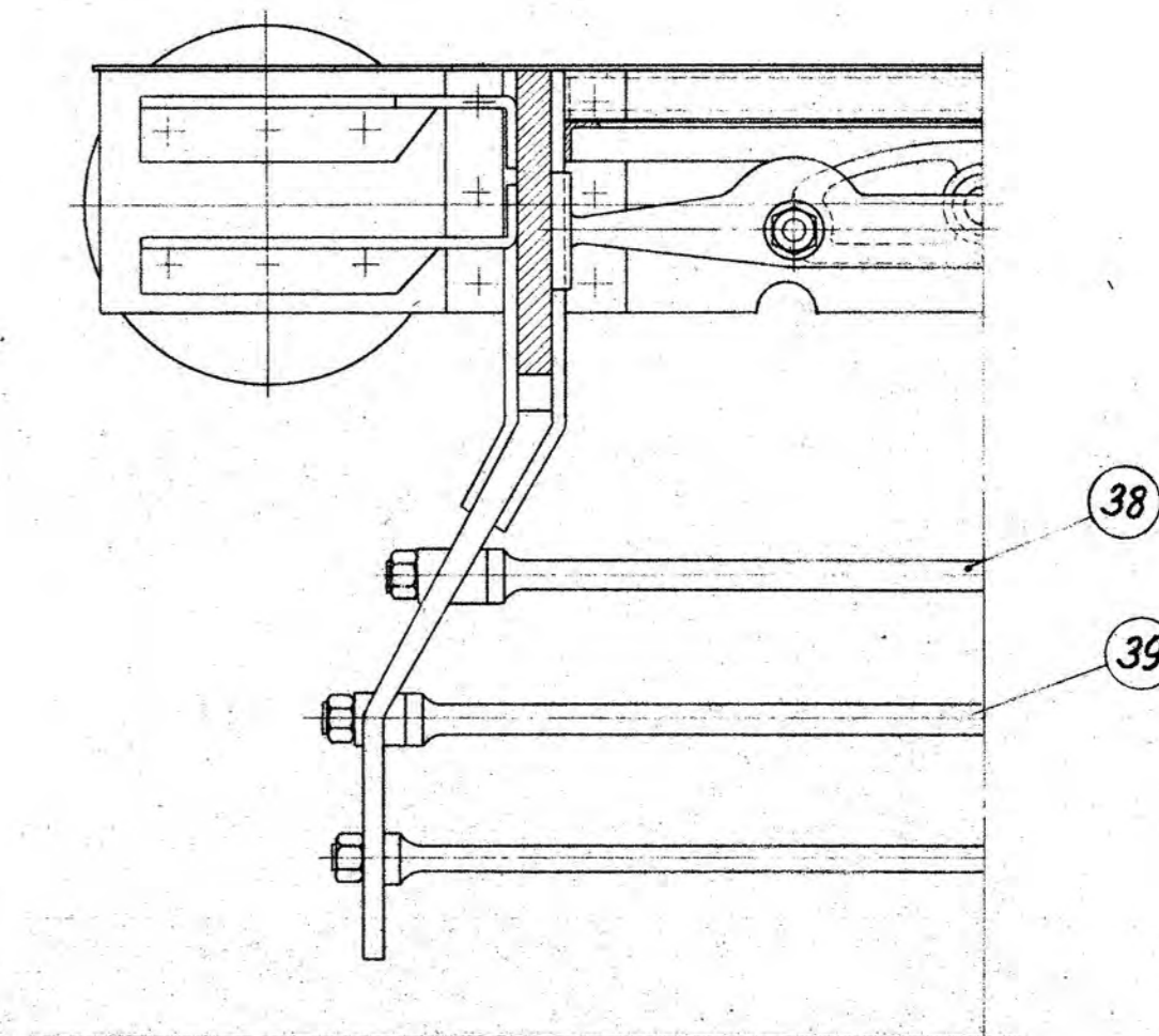
Snit A-A
